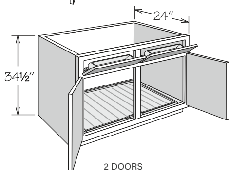
2 DOORS
