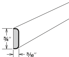
BATTEN
