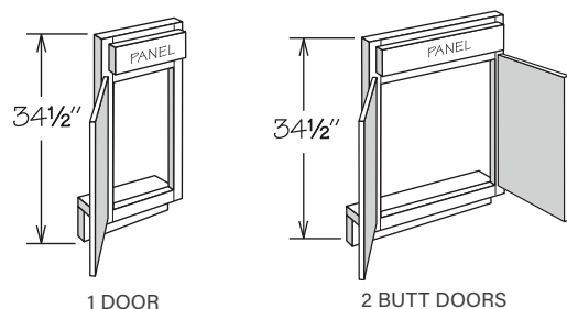
1 DOOR
