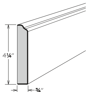
OGEE PILASTER
