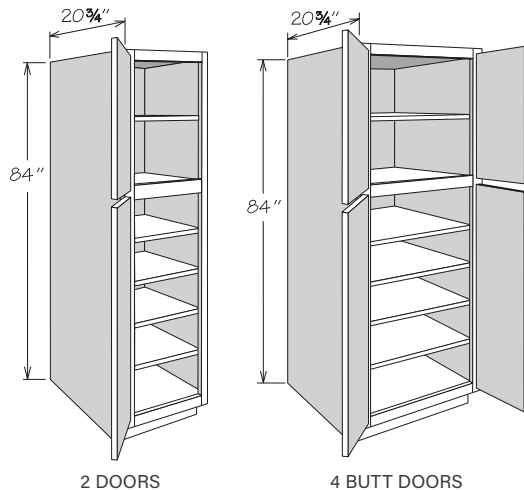
2 DOORS
